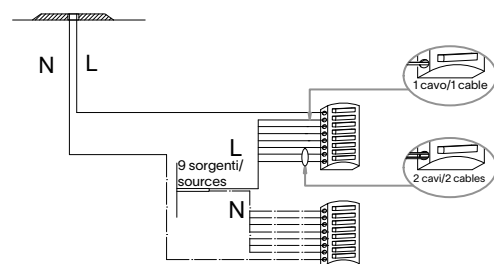
ROSONE D600 9 FORI - schema cablaggio / wiring diagram
