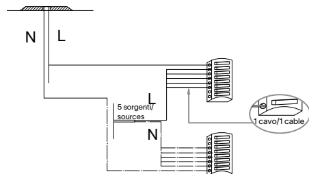
ROSONE D450 5 FORI - schema cablaggio / wiring diagram
