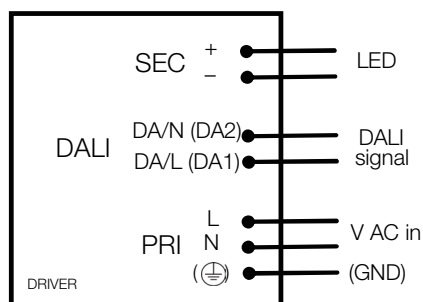
Collegamento DALI DALI diagram
