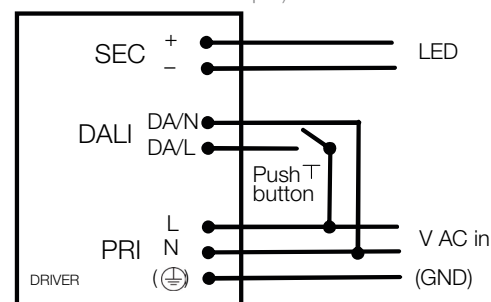
Collegamento PUSH (solo per driver DALI/ Push senza ingresso Push dedicato) PUSH diagram (only for DALI/ Push drivers without dedicated Push input)
